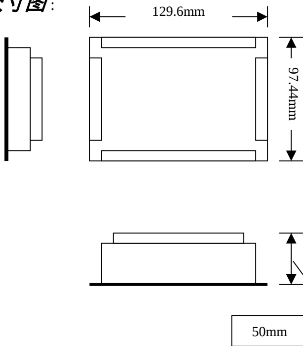
尺寸图:
